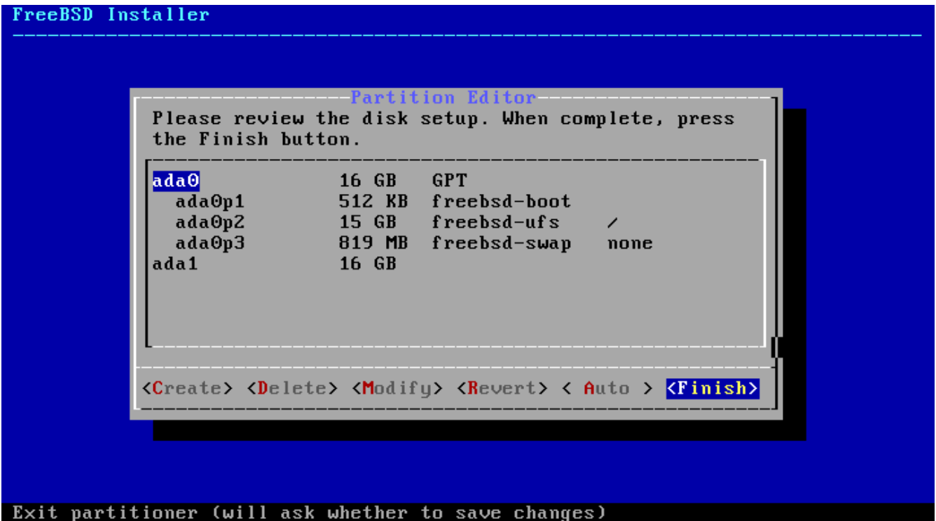
图 70. 检查已创建分区
