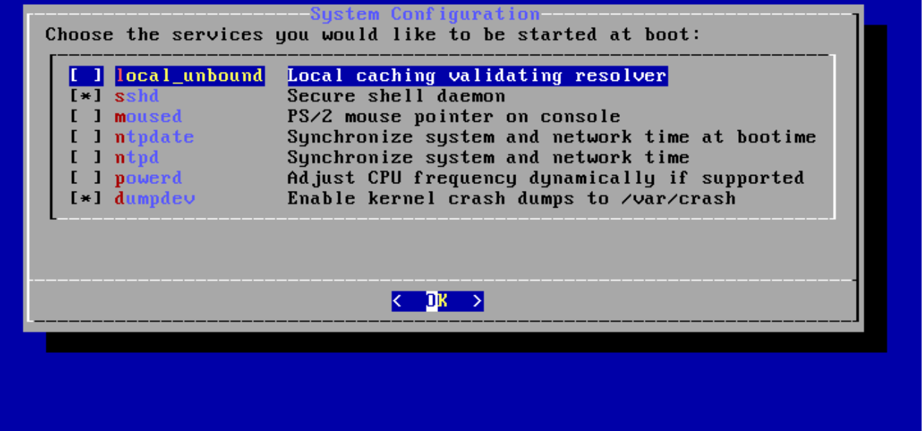
图 95. 选择需要开启的服务
