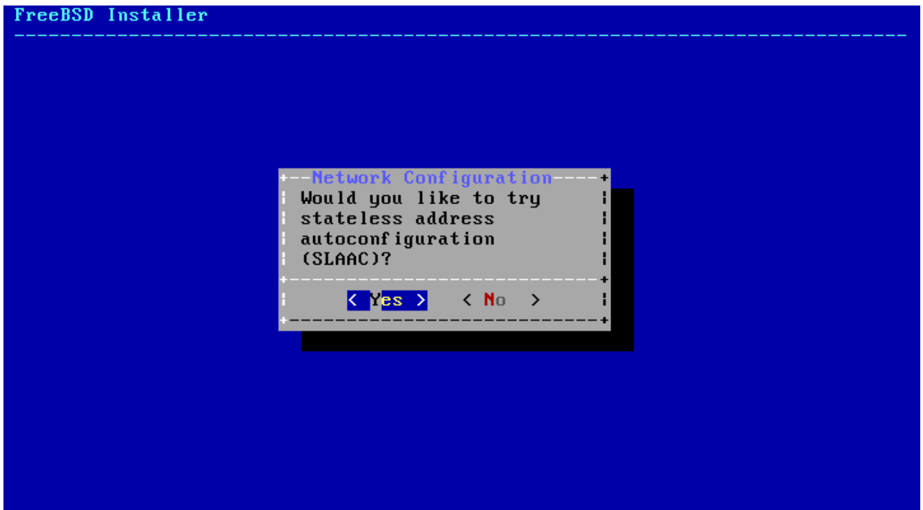
图 87. 选择 SLAAC 配置 IPv6
