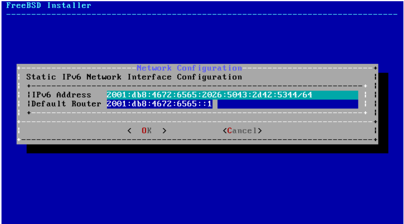
图 88. 静态配置 IPv6
